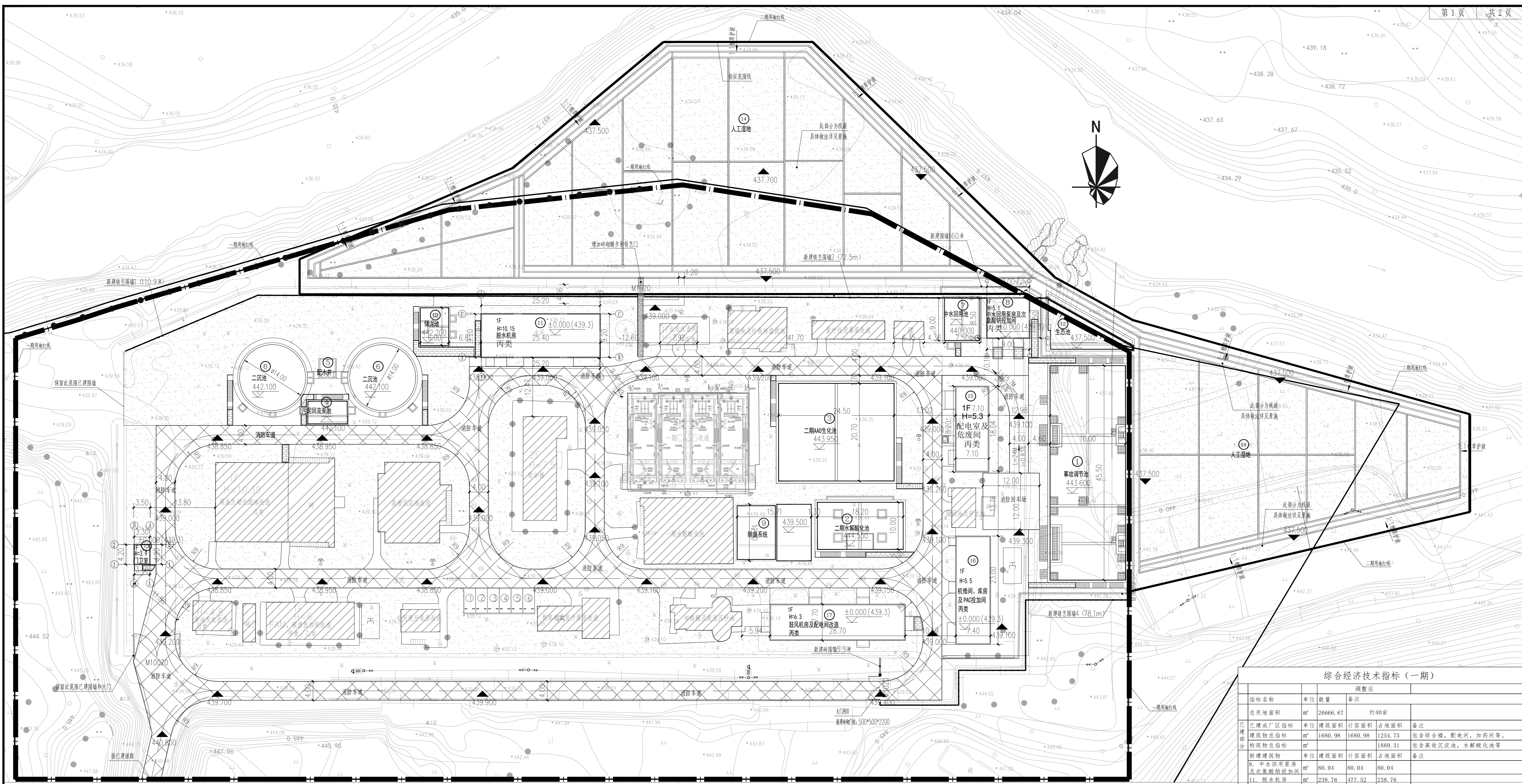
调整后总平面布置图 1:400
