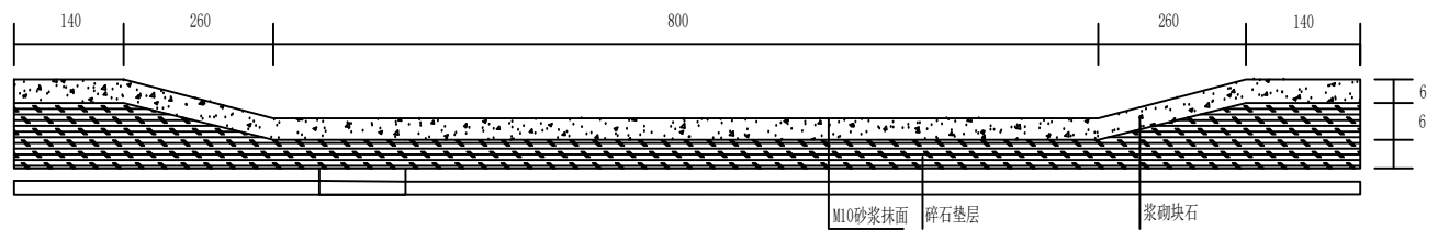
A-A剖视图 1:10
