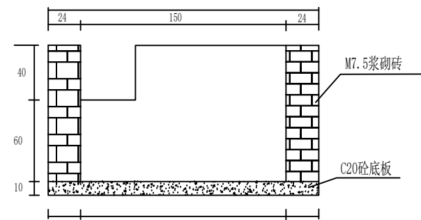
B-B剖面图1:20
