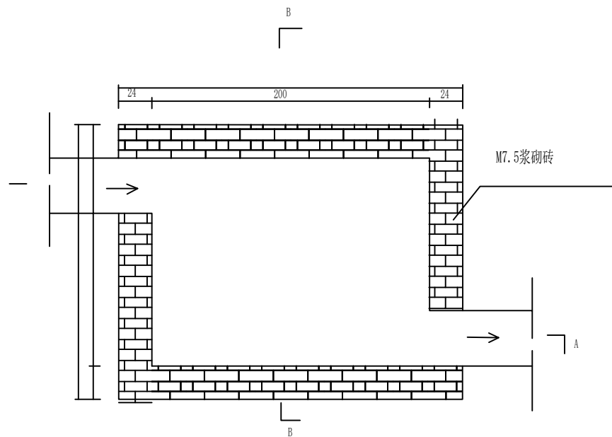
沉砂池平面图1:20
