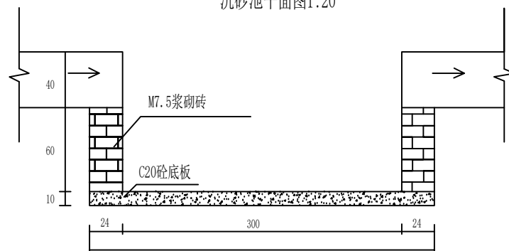
A-A剖面图1:20
