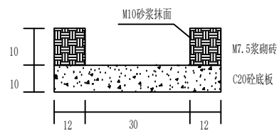
B-B剖视图 1:10
