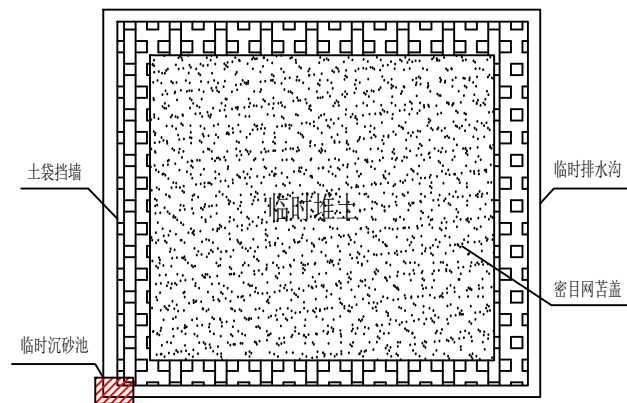
临时堆土区防护平面图 1:100
