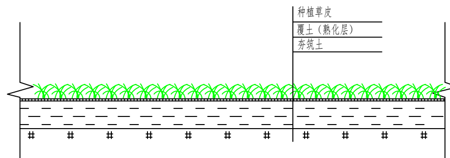
A-A 绿化措施大样图 1:10
