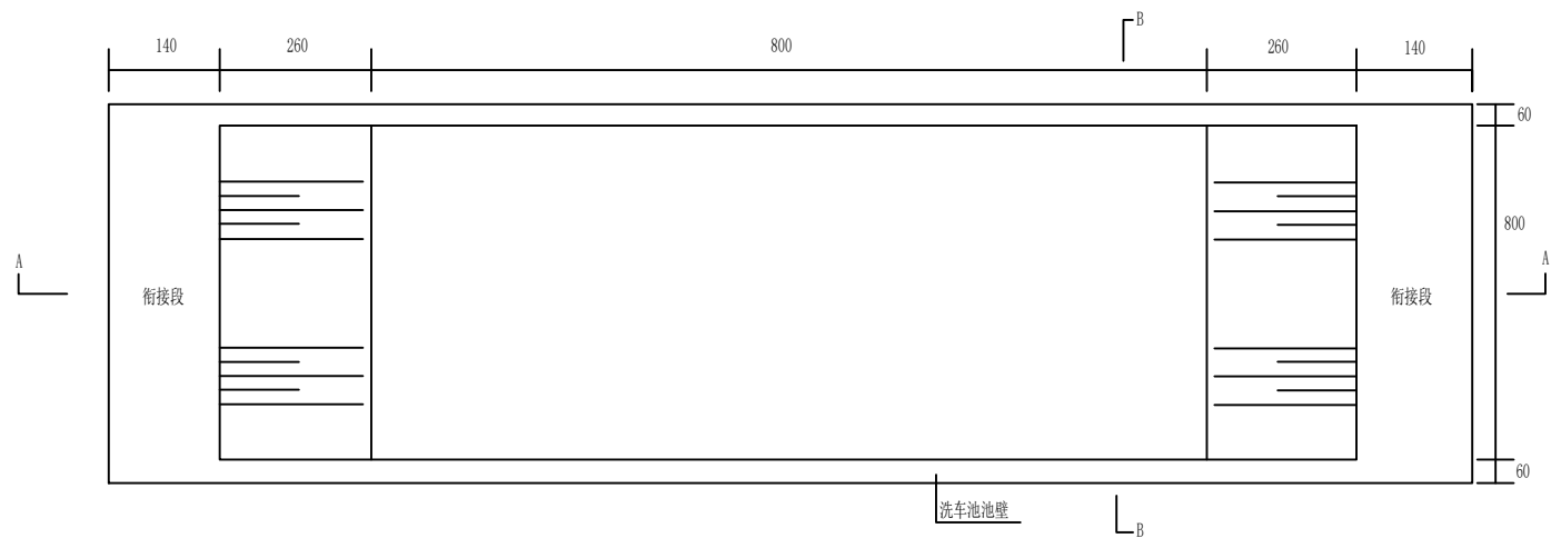
洗车池平面图 1:10
