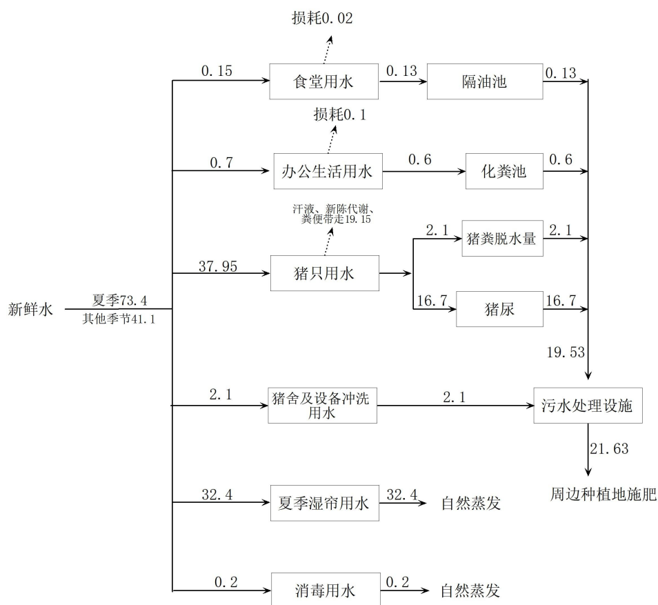
图 4.5-7 项目夏季（最大）水量平衡图 ( \text{m}^3/\text{d} )
